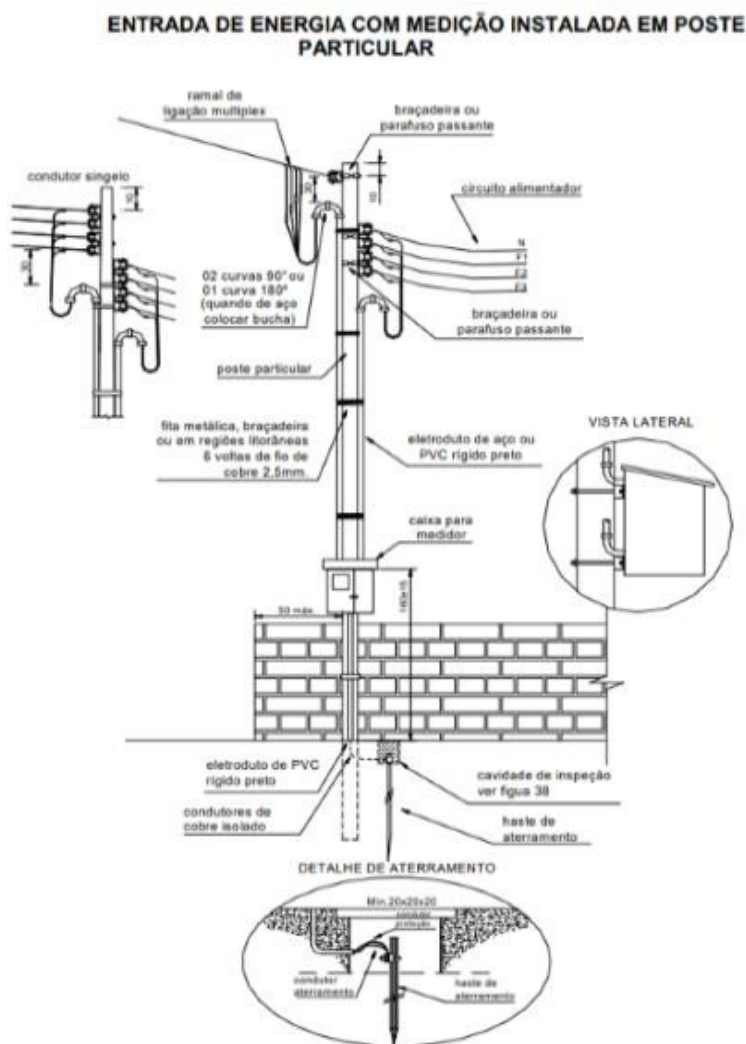
Figura 18- Imagem referência ilustrativa – Elementos entrada de energia.
