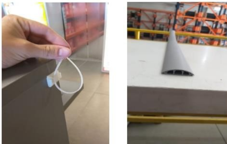
Figura 19- Anilha para organização cabos elétrica e lógica e canaleta de piso para as 03 mesas recepção.
