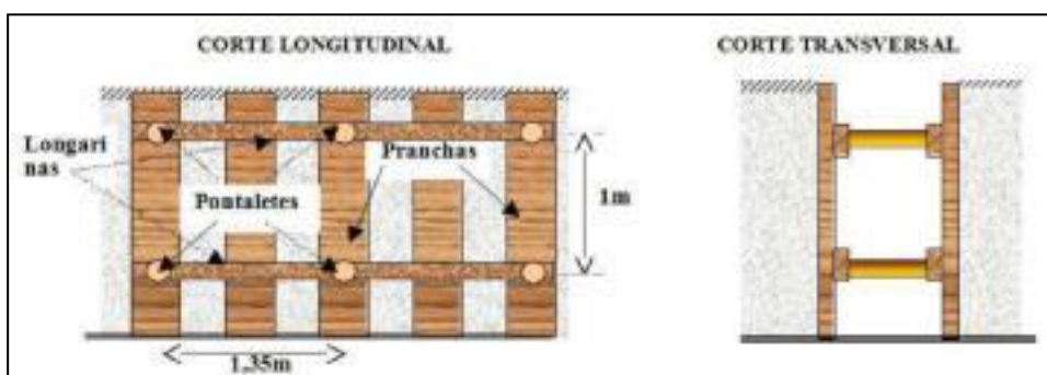
Figura 3 Escoramento descontínuo
